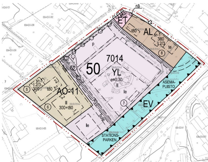
Bild 20. Detaljplaneutkast av planeringsområdet utmed Borghälsvägen
