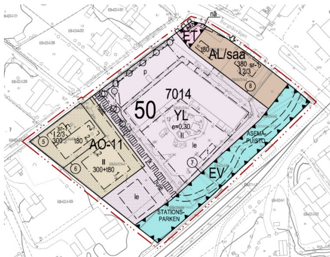
Bild 22. Utdrag ur ett detaljplaneförslag till planeringsområdet vid Borgnäsavägen
