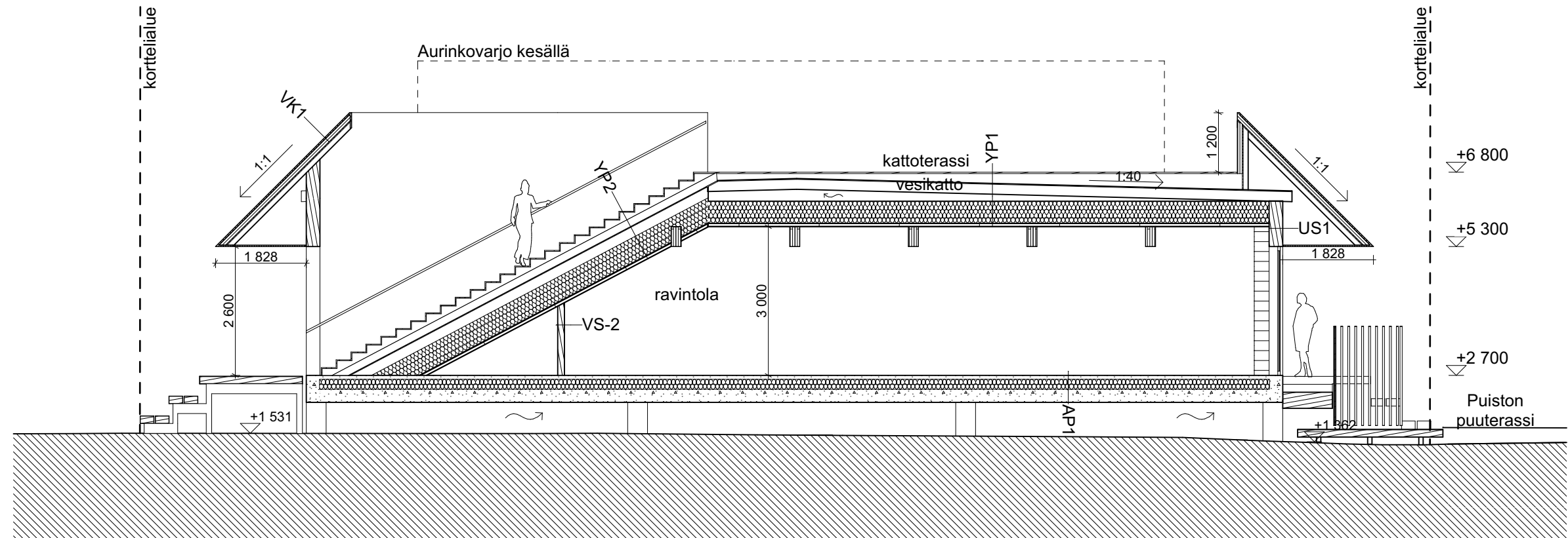
LEIKKAUS B-B
