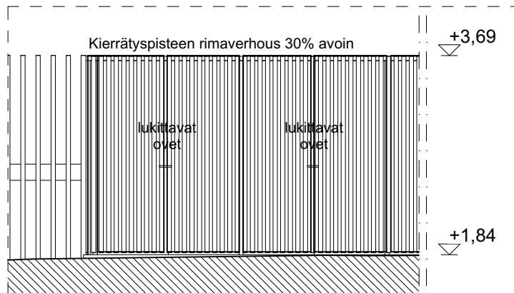
LEIKKAUS D-D: KIERRÄTYSPISTE 1:50
