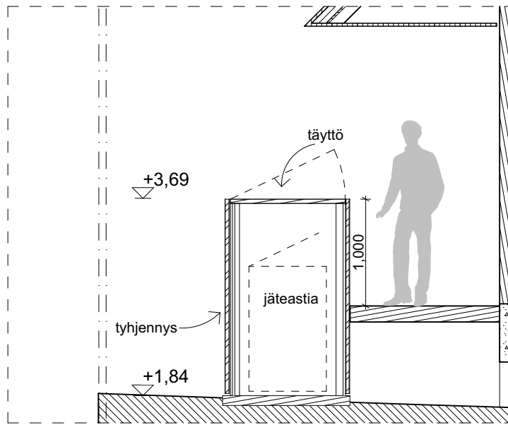
LEIKKAUS C-C: KIERRÄTYSPISTE 1:50
