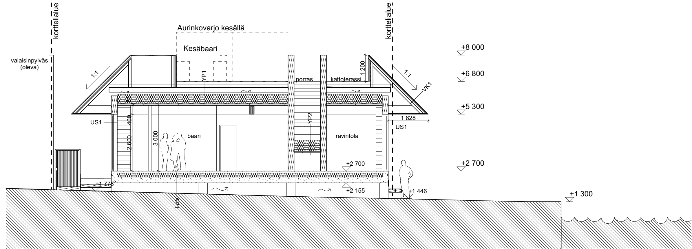
LEIKKAUS A-A
