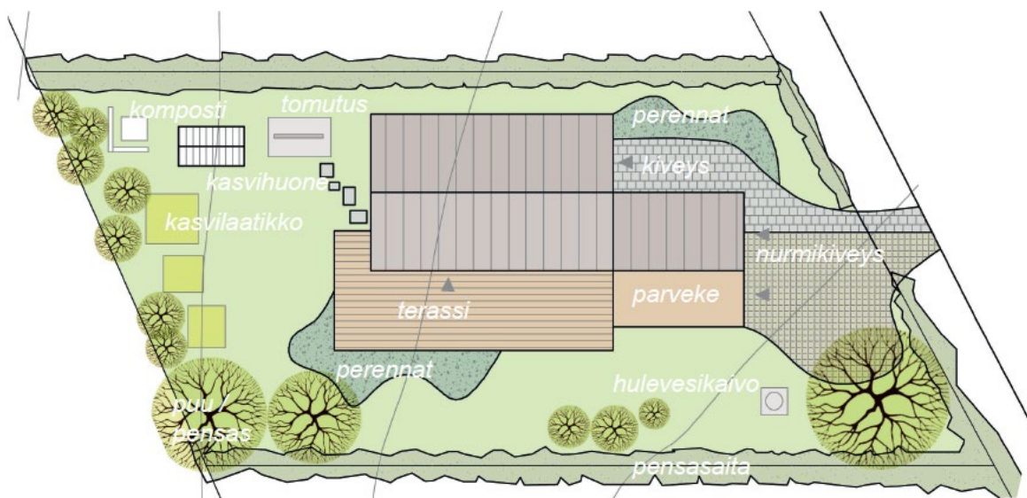
Kuva 3. Esimerkki asemapiirroksesta, jossa on esitetty pihan käyttö. Pysäköintipaikalla on vettä läpäisevä nurmikiveys ja kantava kasvialusta, joka ruokkii pihapuuta. Hulevesikaivo, johon varastoidaan kattosadevedestä kasteluvettä, on pihalla alarinteessä.
